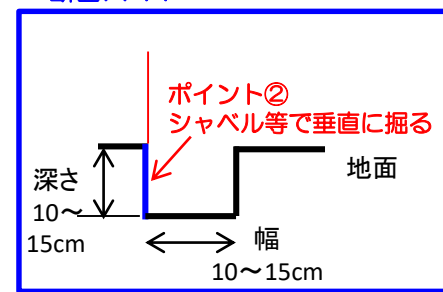
断面A-A
